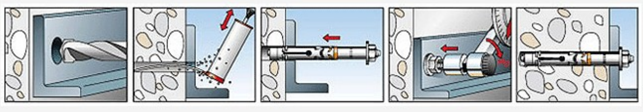
Рис.4, Монтаж анкера.
